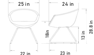
Sled base
