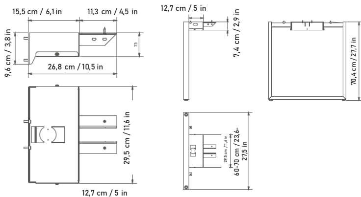
Bajante caja eléctrica lateral costado metálico / Downpipe electrical box side metal side
