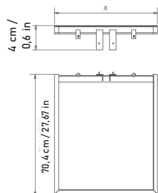
Base rectangular retrocedido derecho / Rectangular base, set back right
