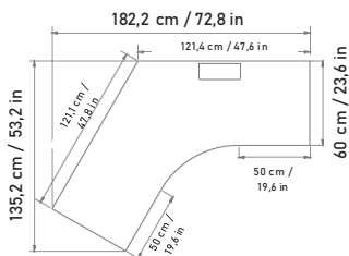
Superficies 120° / 120° surfaces
