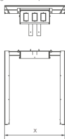
Base caja eléctrica triangular en U / Triangular U-shaped electrical box base
