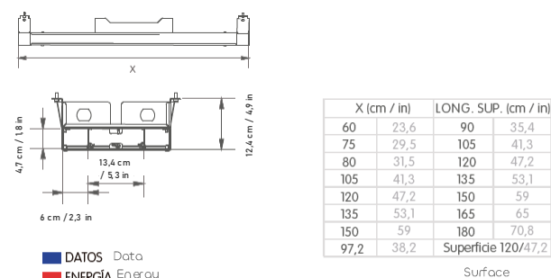
Canaleta doble / Double channel
