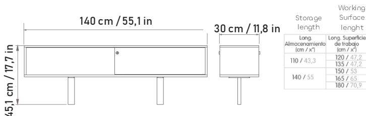
Almacenamiento retorno 150 - archivador 35 / Return storage 150 - filing cabinet 35
