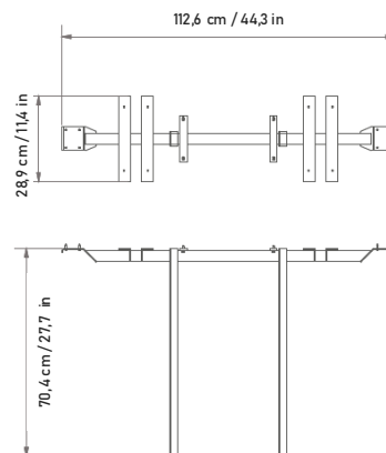
Base central doble / Double central base
