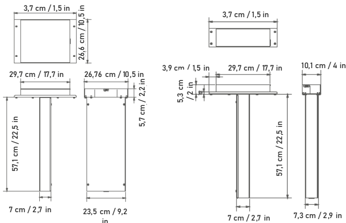
Bajante doble / Double downpipe
