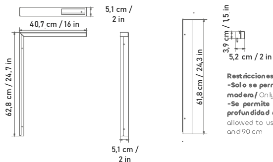
Bajante caja eléctrica lateral costado metálico / Downpipe electrical box side metal side
