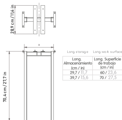
Base central doble / Double central base
