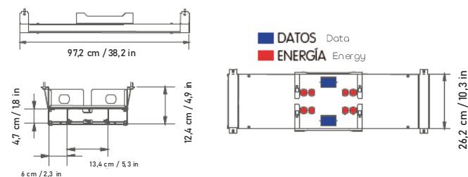
Canaleta doble 120° / Double channel 120°
