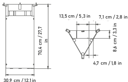
Caja eléctrica lateral costado madera / Electrical box on the side of the wooden side panel
