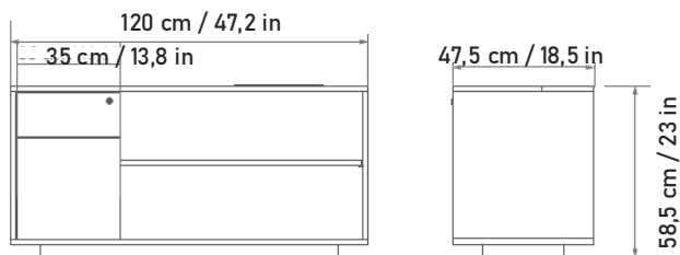
Almacenamiento retorno 120 - archivador 35 / Return storage 120 - filing cabinet 35
