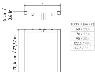
Base cua drada / Square base
