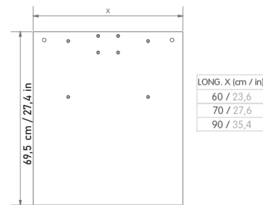
Base escritorio madera / Wooden desk base
