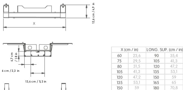
Canaleta doble ensamble viga / Double beam assembly channel
