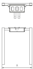
Base caja eléctrica cuadrada / Square electrical box base
