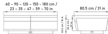
Sin espaldar / Without backrest
